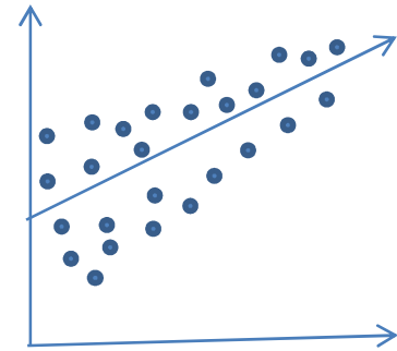
شكل (1-C) يوضح حالة عدم ثبات التباين مع زيادة في المتغير التوضيحي ( x_i )
