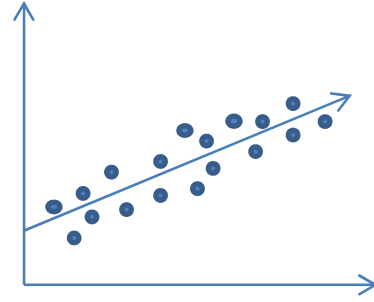
شكل (1-A) يوضح حالة ثبات التباين التباين
