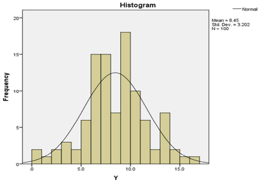
الشكل (2) يوضح توزيع بيانات المتغير المعتمد (Y)
