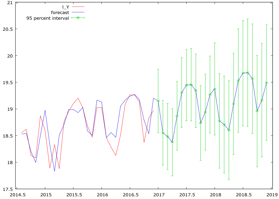
الشكل (8-3) يمثل القيم التنبؤية لسلسلة كمية الطاقة الكهربائية الضائعة وفق إنموذج SARIMA(0,1,1) \times (0,1,1)_{12}
