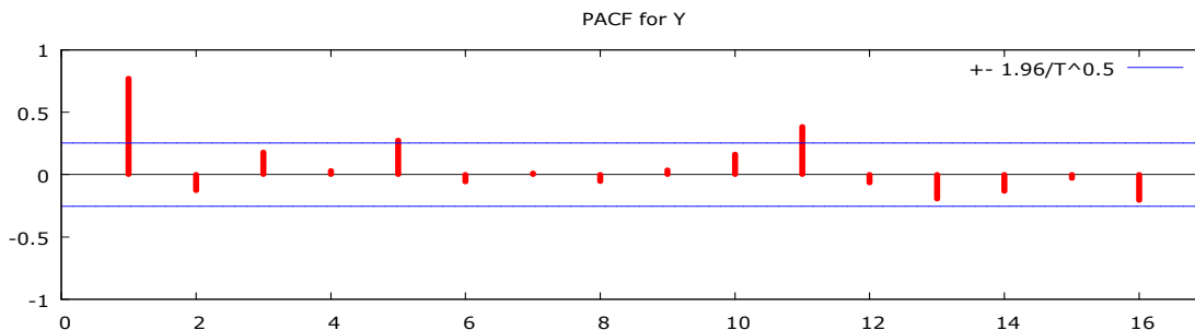
الشكل (3-2) - ب دالة الارتباط الذاتي الجزئي PACF للبيانات
