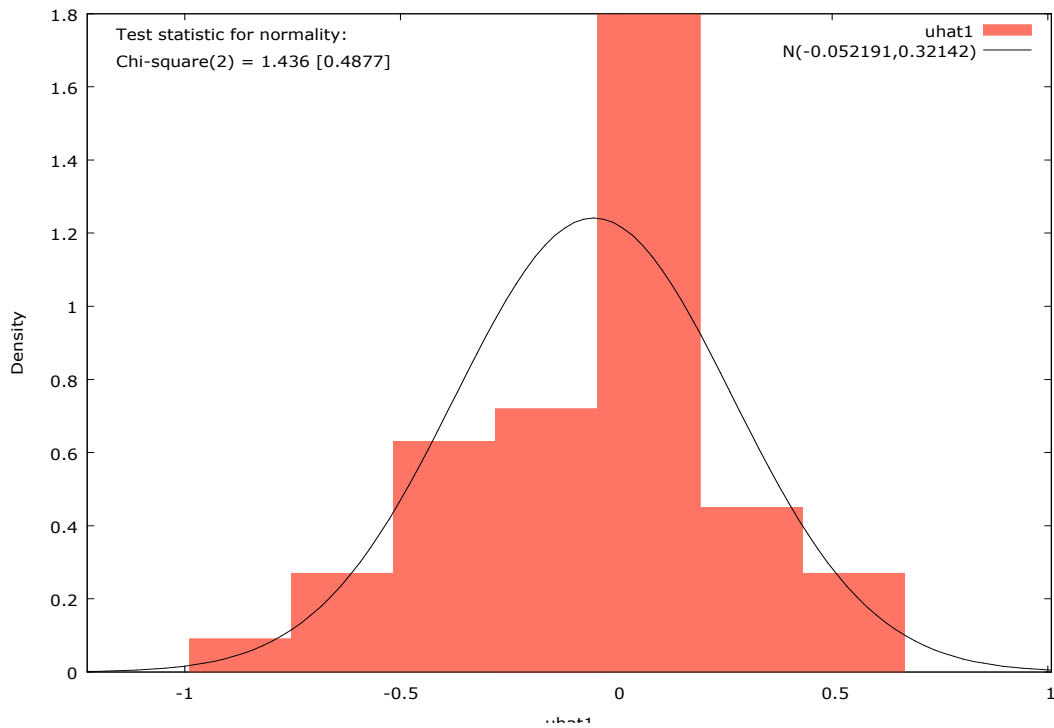
شكل(6-3) يوضح التوزيع الطبيعي للبقايا
