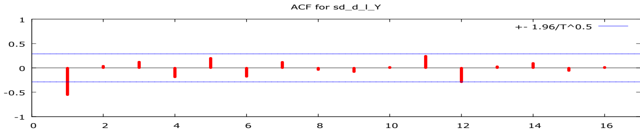
الشكل (4-3)- أ دالة الارتباط الذاتي ACF لسلسلة الفروق واللوغاريتم الطبيعي
